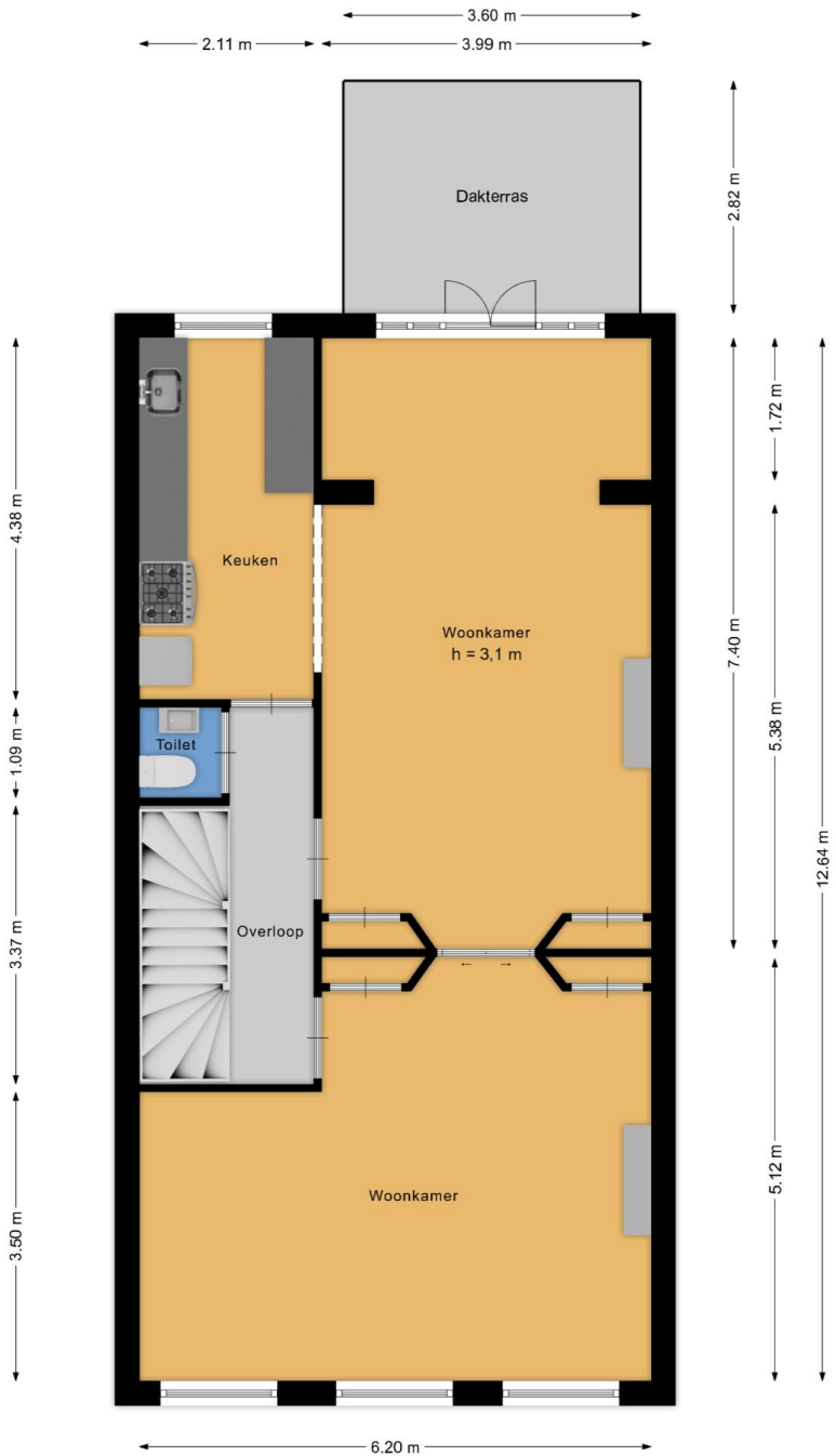
1e verdieping
